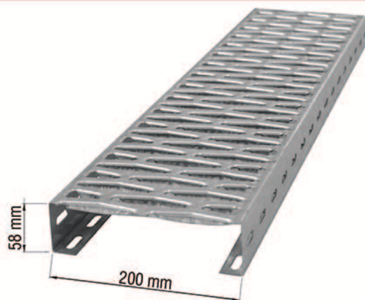
GRIGLIATO GP ABA/GP200 sez. 200x58 mm zincato barre L.350 cm
