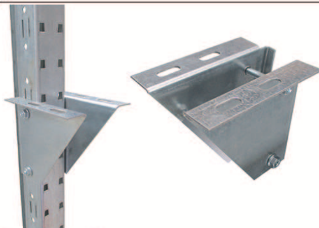
STAFFA SOPPALCO ET.CSPS/C zincato
