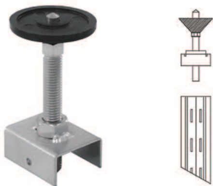
TAPPO A SOFFITTO PER MONTANTE M35
