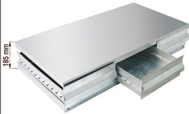
BLOCCO A 3 CASSETTI ET.B/9640/Z L.96 x P.40 cm zincato BLOCCO A 3 CASSETTI ET.B/9650/Z L.96 x P.50 cm zincato DIVISORIO PER CASSETTO ET.B/DIV/Z L.32 cm zincato
